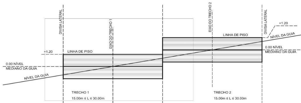
CORTE ESQUEMÁTICO
