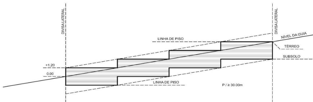
CORTE ESQUEMÁTICO
