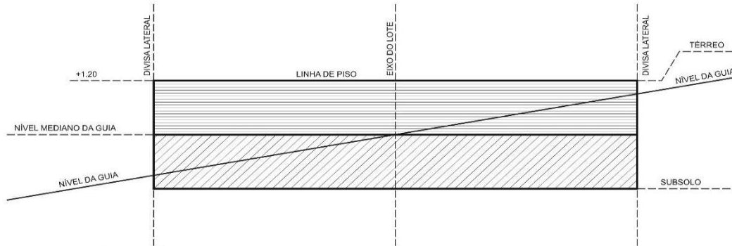
CORTE ESQUEMÁTICO
